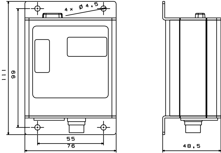
智能数字振动送料控制器SDVC20-S外形尺寸
