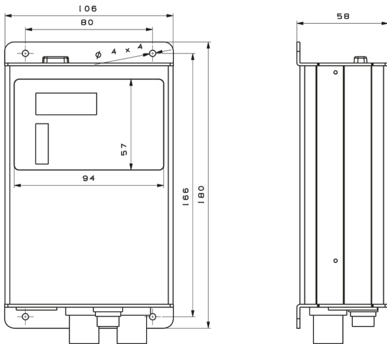
智能数字振动送料控制器SDVC20-L外形尺寸
