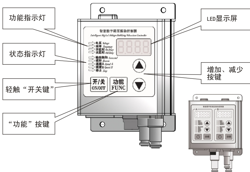
SDVC22 双数字调压振动送料控制器
