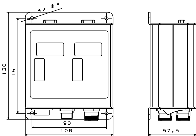
智能数字振动送料控制器SDVC22外形尺寸
