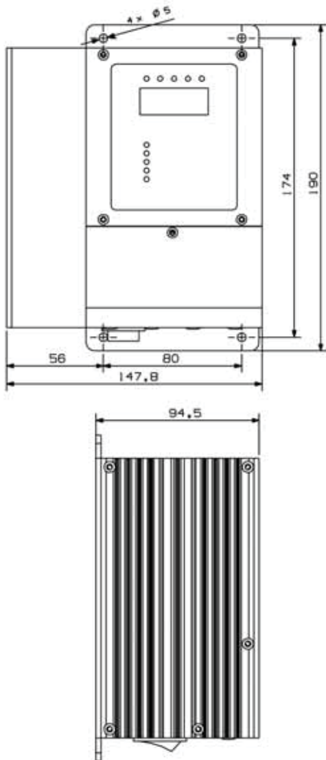
SDVC31-L、SDVC31-XL电磁调频振动送料控制器外形尺寸
